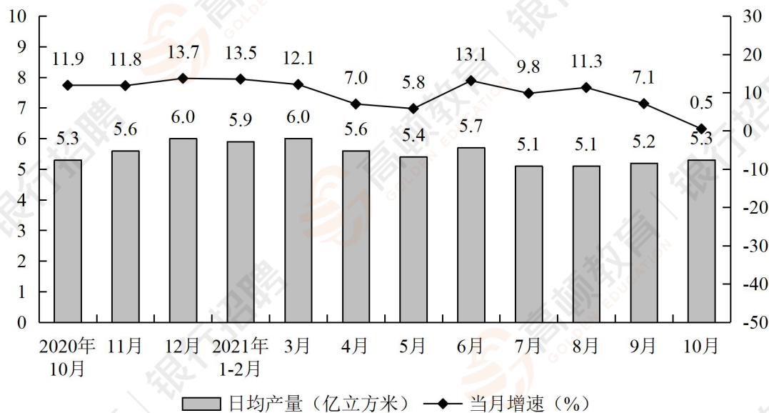
图 1 规模以上工业天然气产量月度走势图
